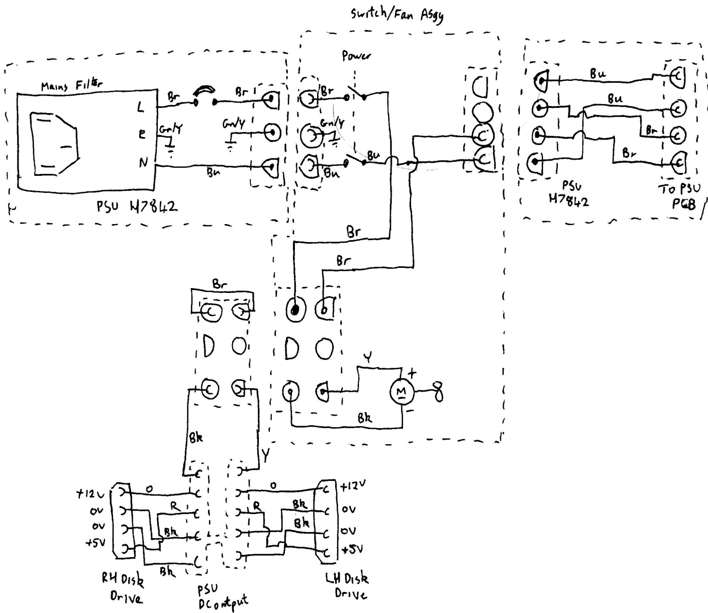
Rainbow PSU Wiring
